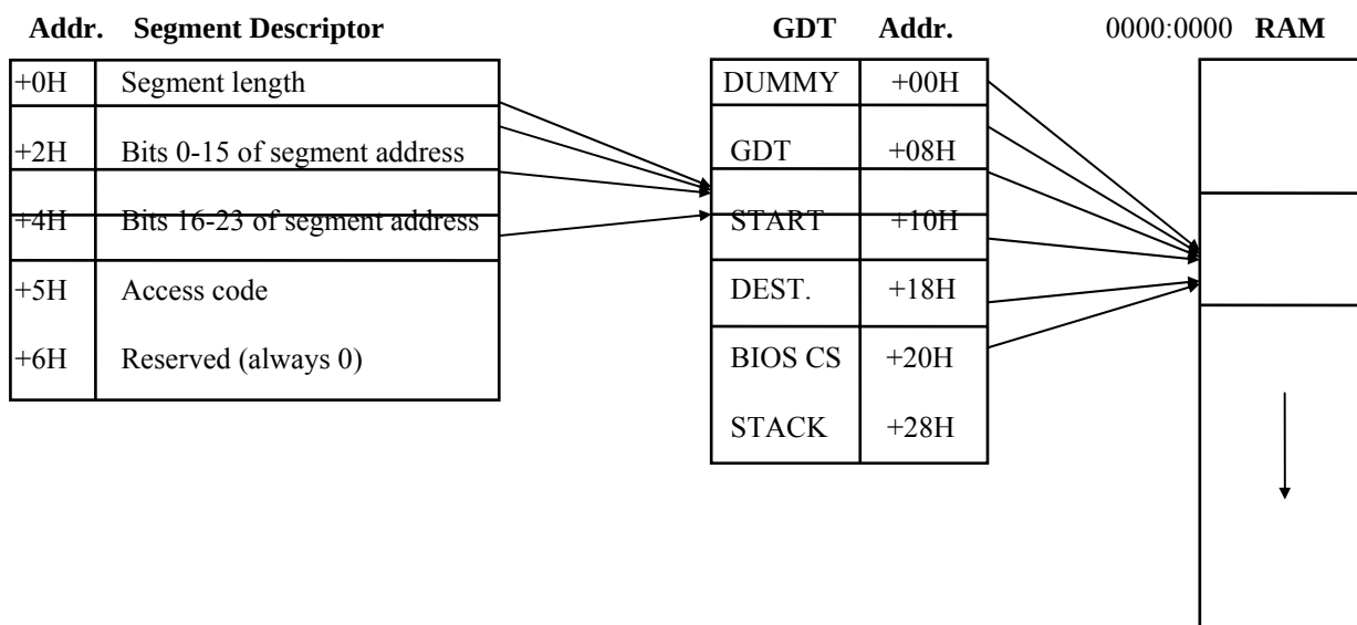
شکل ۱۲-۲: ساختار توصیف گر قطعه از نظر وقفه‌ی 87H
